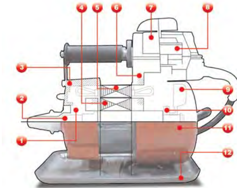
Рис.2. Электродвигатель вибраторов ВЭ-75, ВЭ-11-3, ВЭ-11-7А, ВЭ-11-6А-1,6, ВП-75, ВП-75 1 – муфта сцепления; 2 – шпиндель; 3 – щит передний; 4 – ротор; 5 – статор; 6 – щит задний; 7 – крышка; 8 – выключатель пакетный; 9 – вентилятор; 10 – подшипник; 11 – кожух; 12 – основание.
